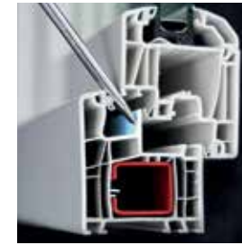
Mittelsteg für hohen Aushebelschutz
