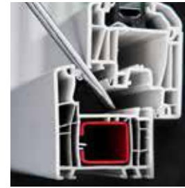
Vergleichbare Fenster ohne Mittelsteg
